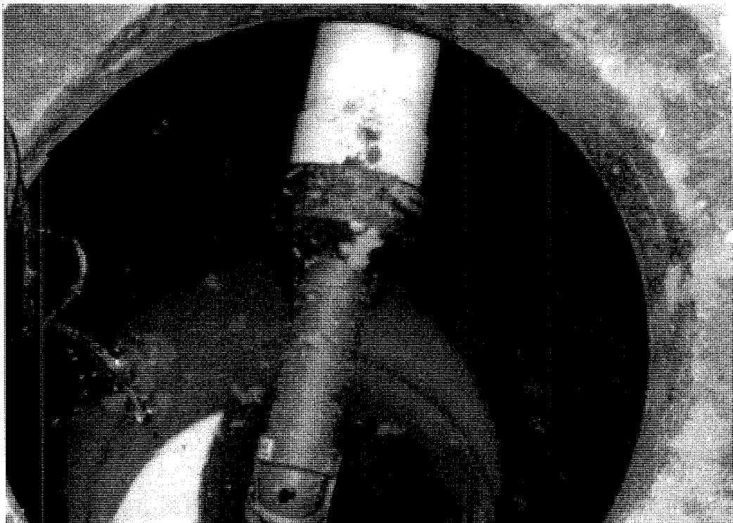
Photo 48 - sites 001 à 046 - deuxième compartiment de la fosse septique muni d'une pompe
