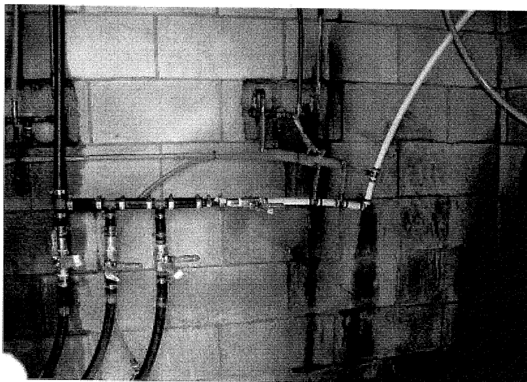
Photo 15 - bloc sanitaire 2 - conduites servant au chauffage radiant utilisées pour l'eau potable
