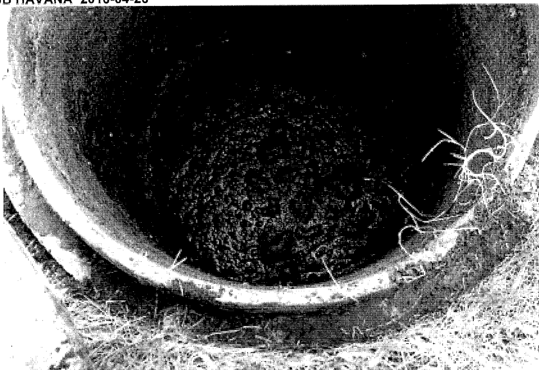
Photo 52 - fosse septique de l'hôtel - présence de boues dans le deuxième compartiment
